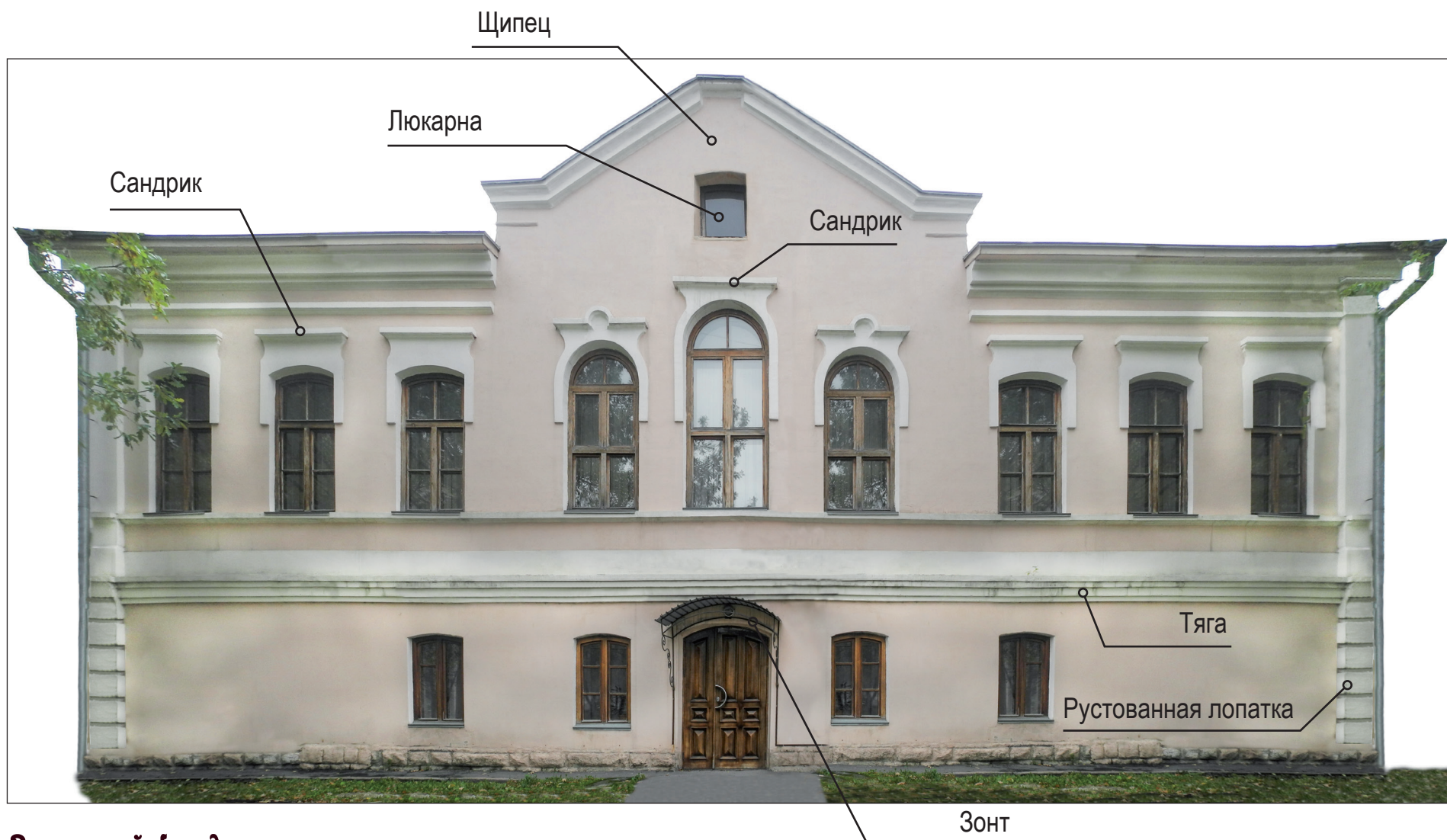
Восточный фасад
