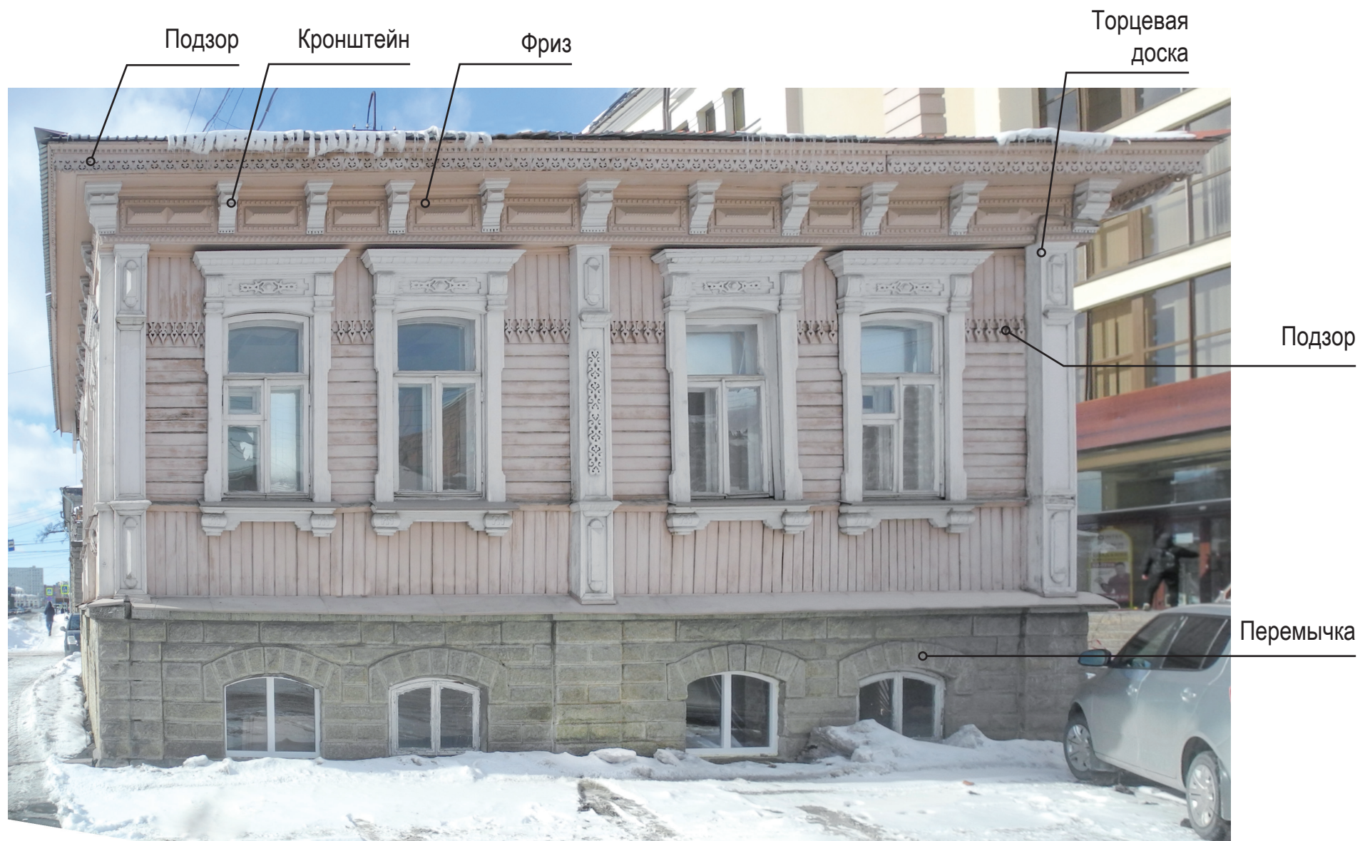
Восточный фасад
