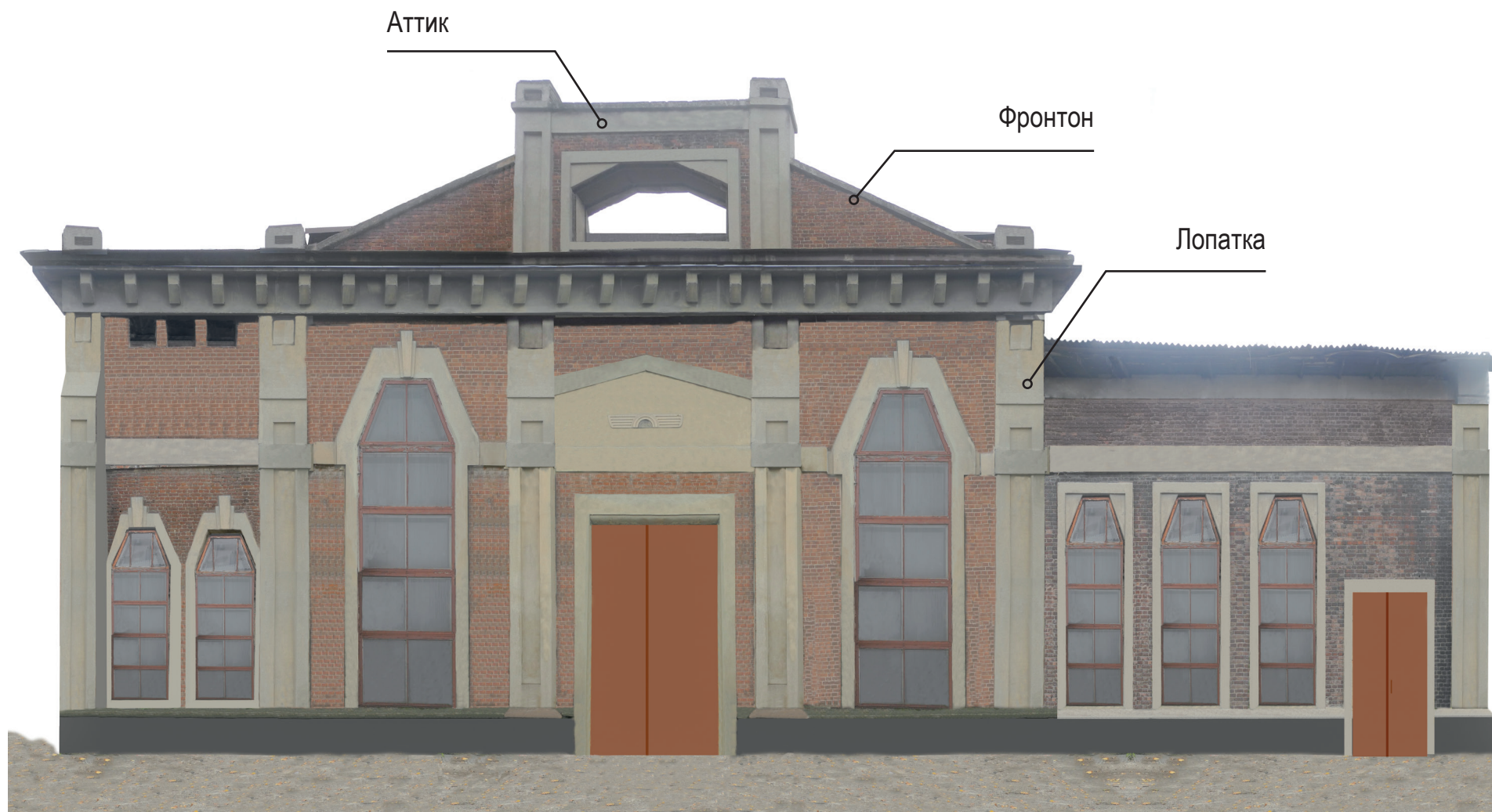
Восточный фасад
