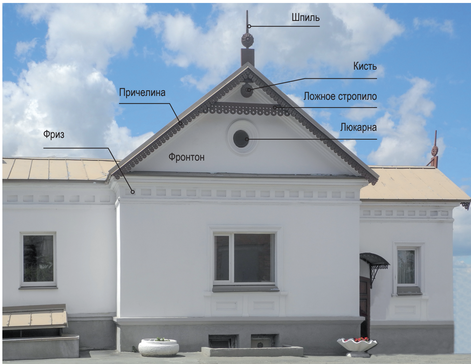
Восточный фасад
