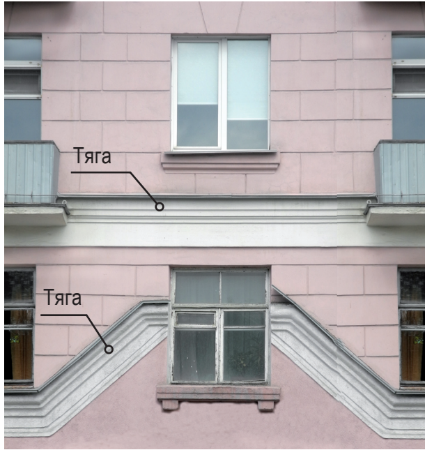
Фрагмент фасада
