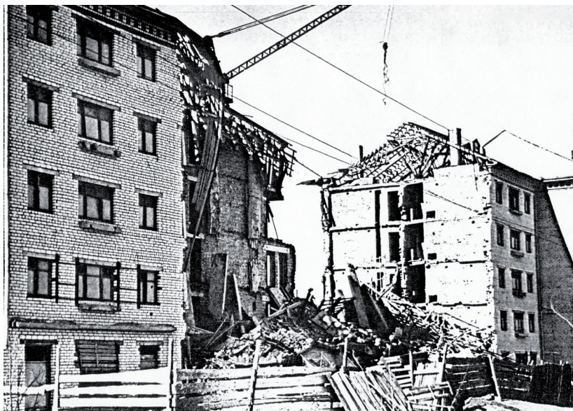
Рис. 5.1. Вид строящегося здания после обрушения
